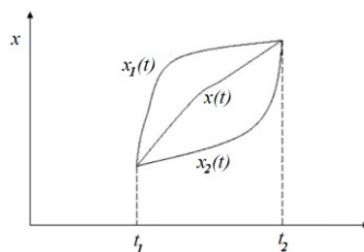
Figura 3 Camí òptim entre dos punts fixos i dues possibles deformacions infinitessimals del camí (exagerades)
