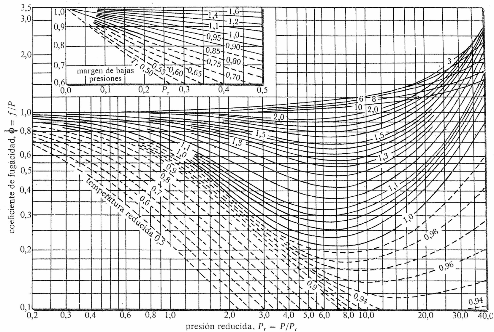
Figura 14-5. Coeficientes de fugacidad de los gases. Basado en datos tomados de B. W. Gamson y K. M. Watson, Natl. Petrol. News, Tech. Sec. 36, R623 (Set. 6, 1944).
